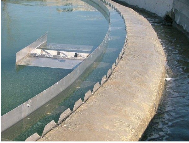
(ÇÖKTÜRME HAVUZU V SAVAK VE DALGIÇ PERDE)
